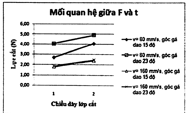
Hình 4. Mối liên hệ giữa chiều dày lát cắt và lực cắt
