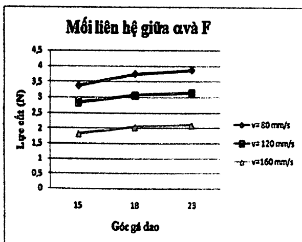
Hình 2. Mối liên hệ giữa góc gá dao và lực cắt
