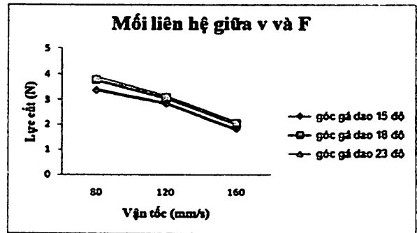
Hình 3. Mối liên hệ giữa góc vận tốc cắt và lực cắt
