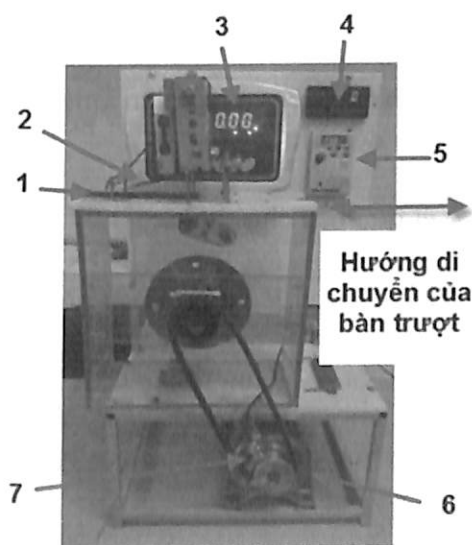
Hình 1. Mô hình thí nghiệm:
